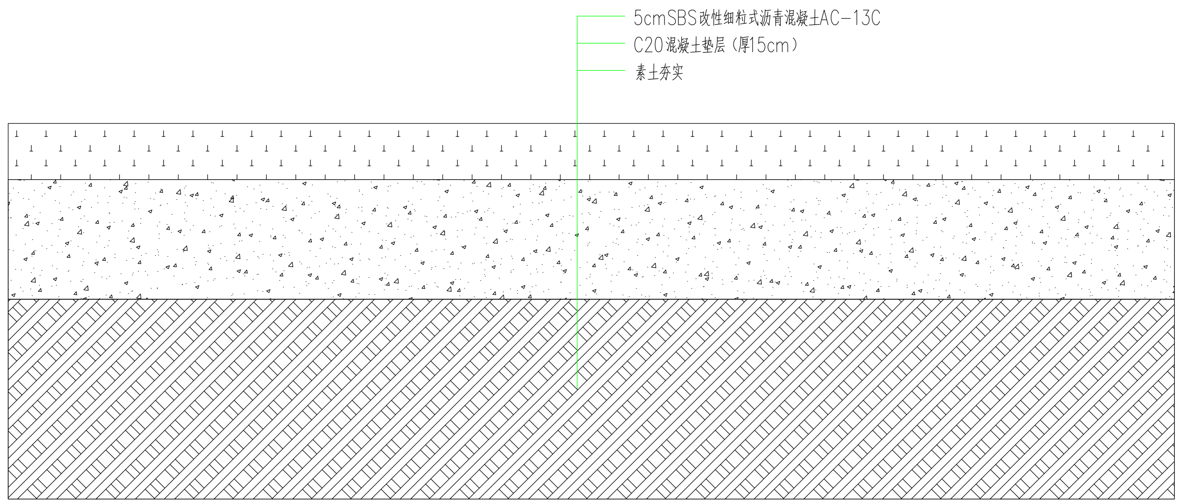
院坝 250m 2 沥青混凝土断面图
