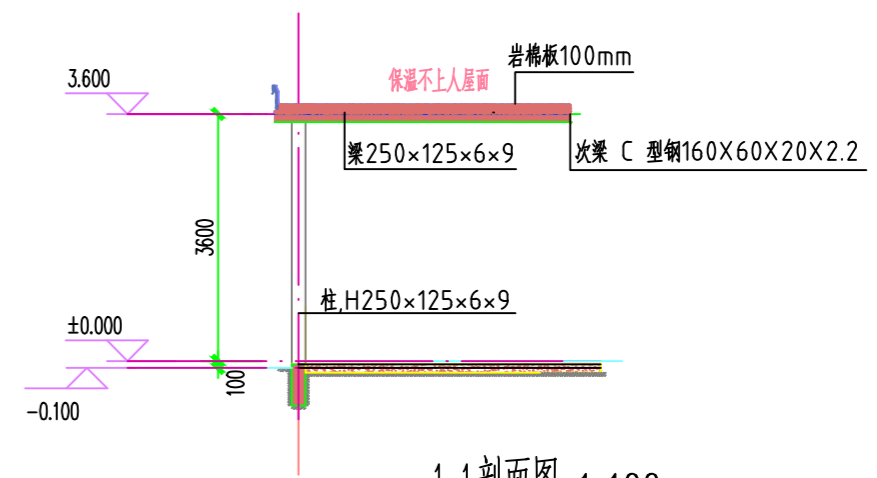
1-1剖面图 1:100
