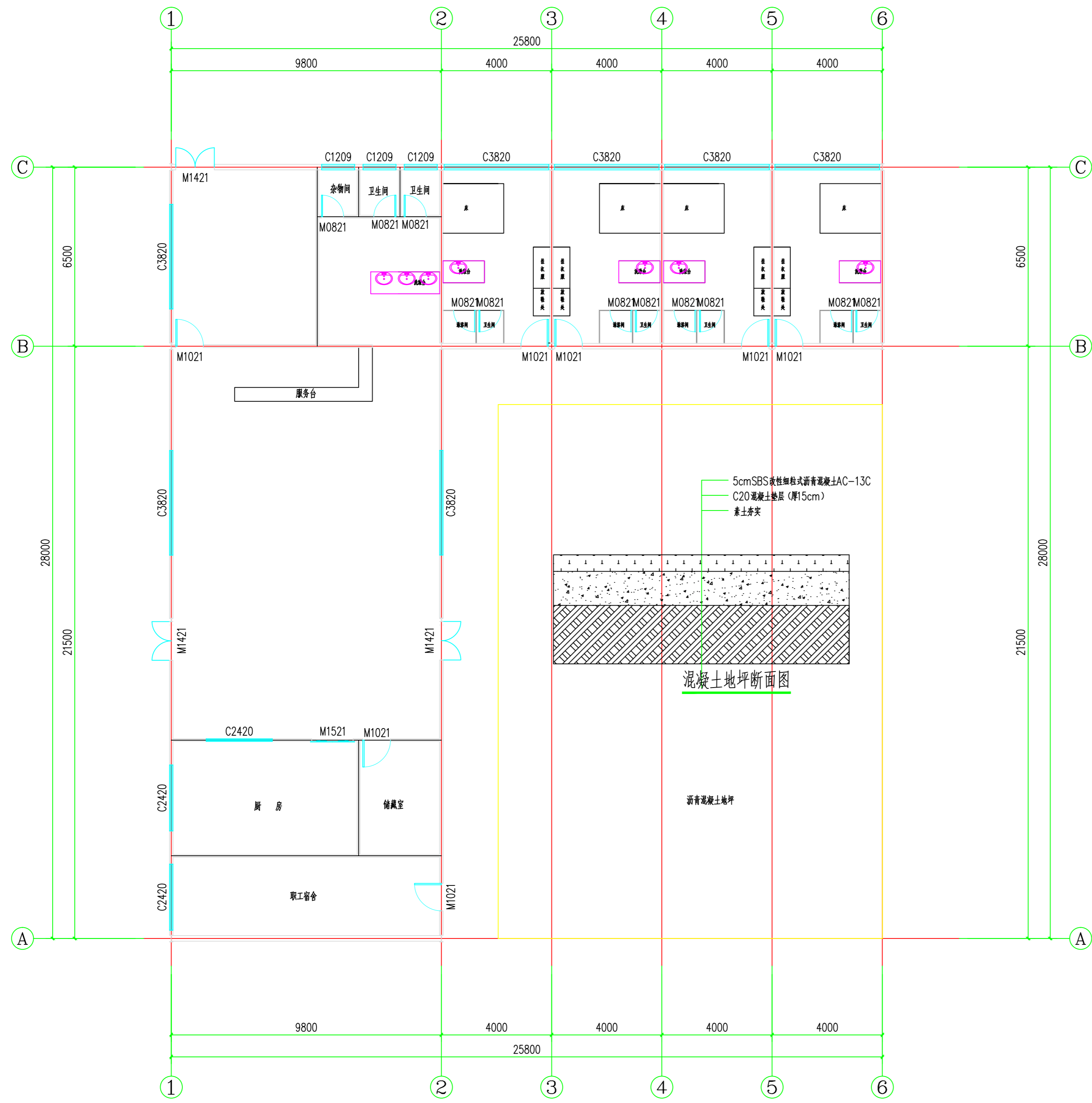
一层平面图 1:100
