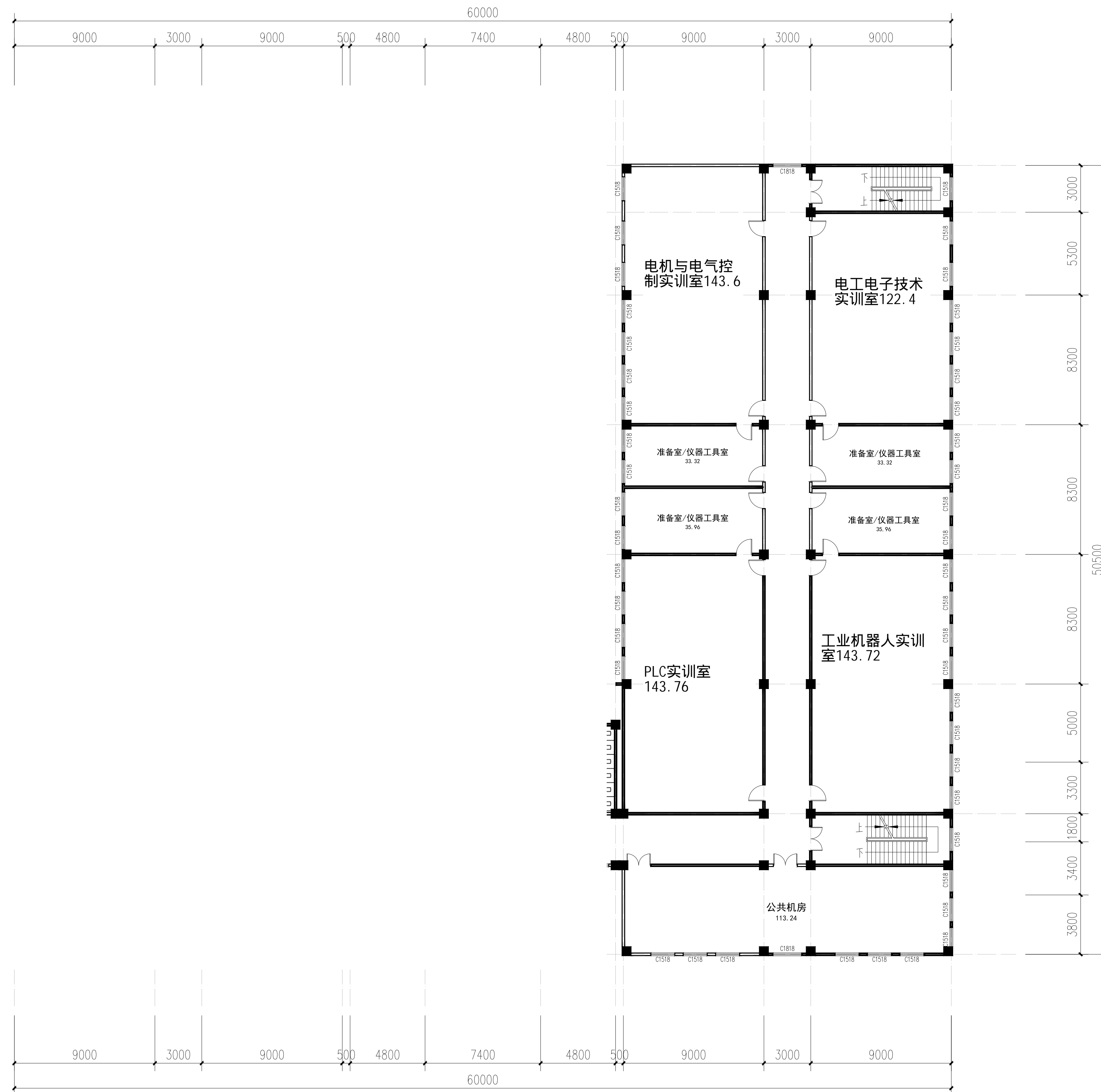
二层平面图 1:100 本层面积为：2310.02平方米
