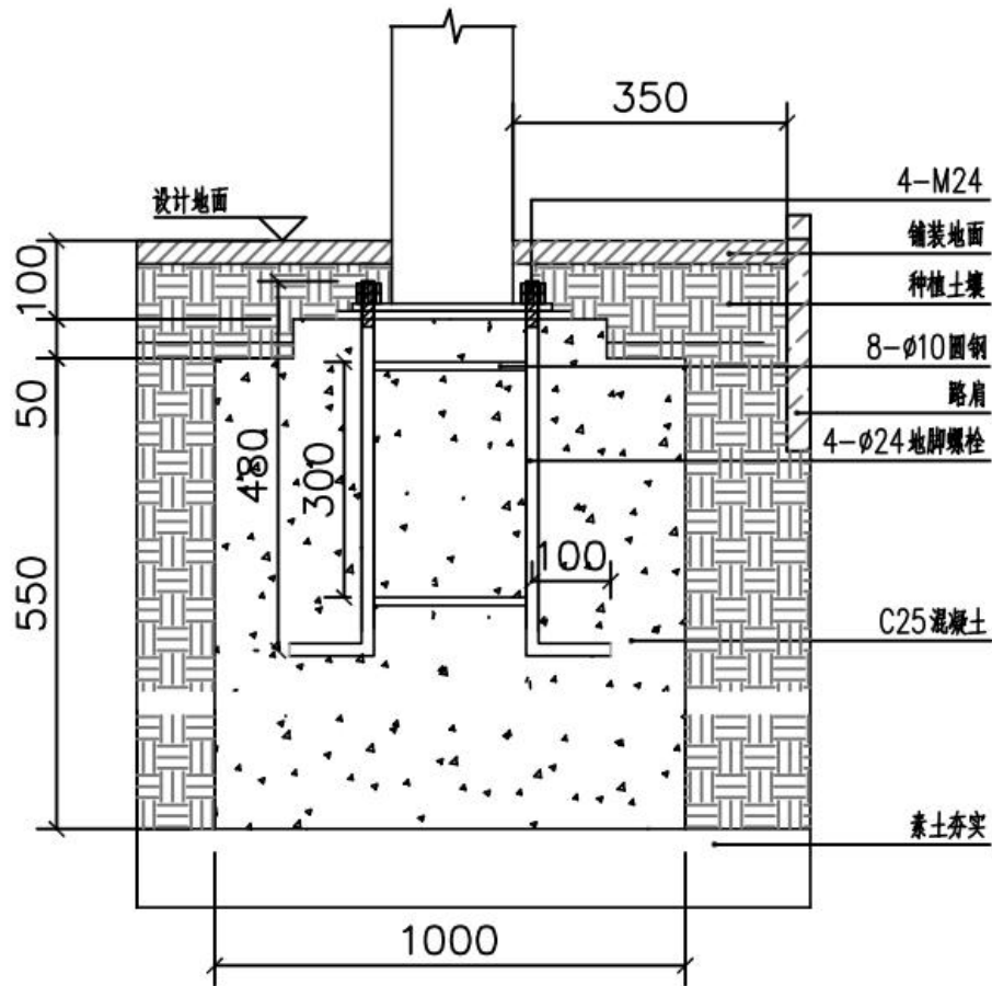
基础安装做法示意图
