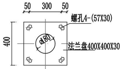
法兰盘大样图 1:100
