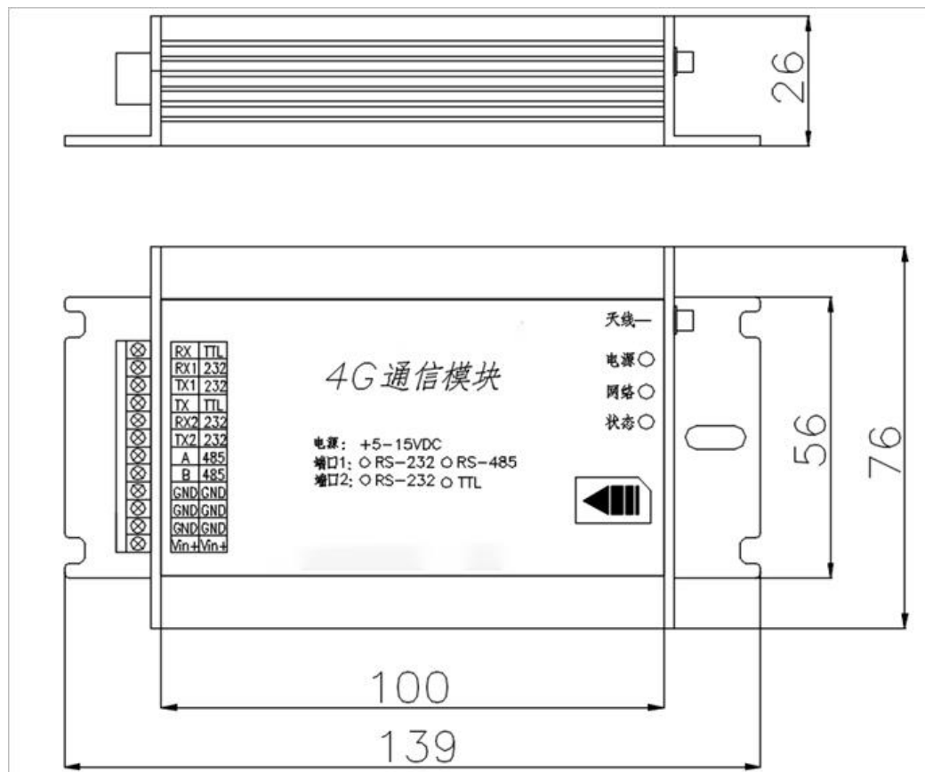
4G 通信模块外形尺寸（单位：mm）
