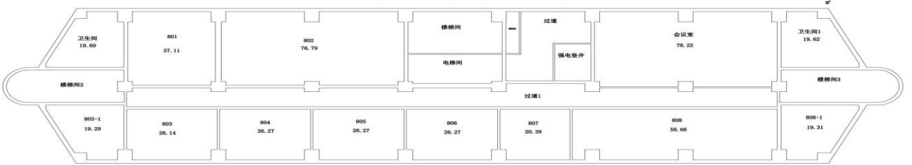
八层平面图 1:100 建筑面积: 739.13m 2
