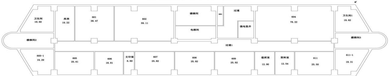
六层平面图 1:100 建筑面积: 739.13m 2 单位名称: 新疆维吾尔自治区科学技术馆 地址: 乌鲁木齐市沙依巴克区新医路686号 作业单位: 新疆金罗盘测绘有限公司
