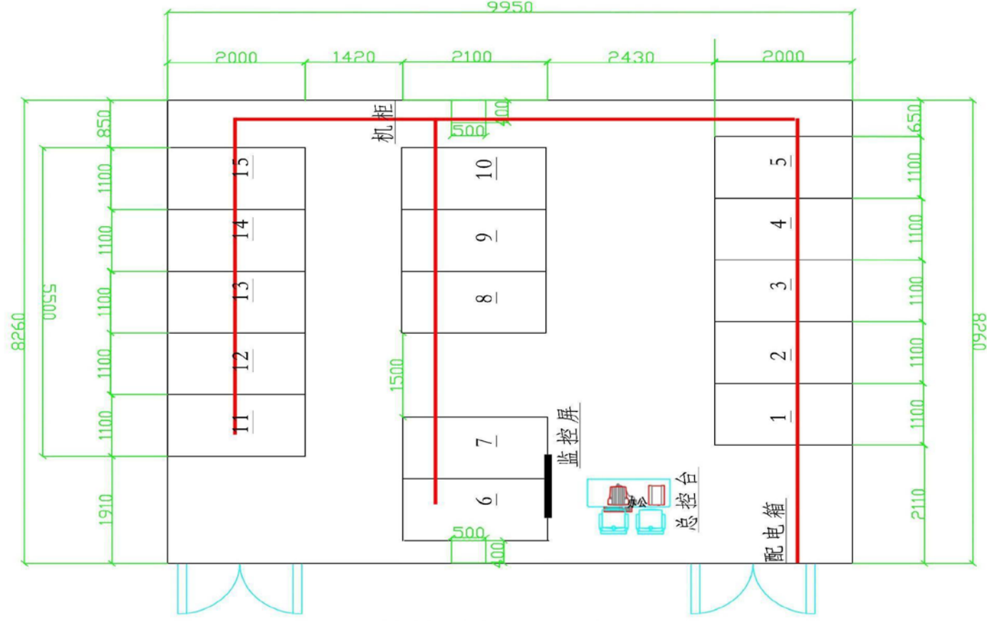
新校区新建平面图 图上尺寸单位mm
