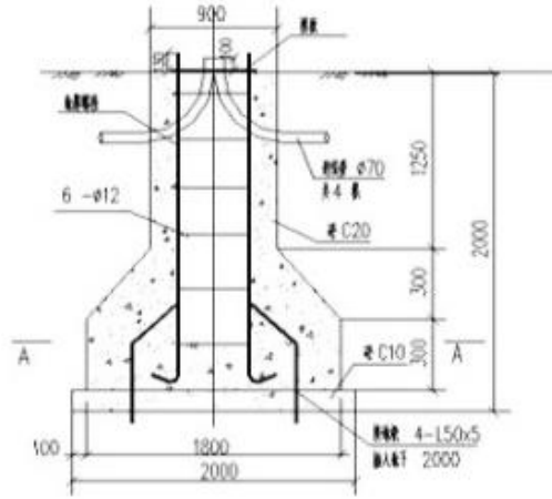
14米中杆灯杆基础图
