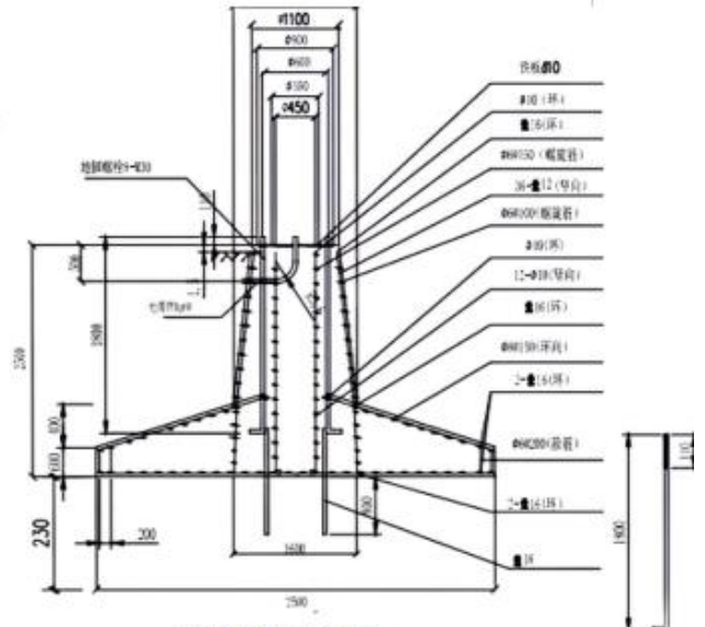
18米中杆灯杆基础图
